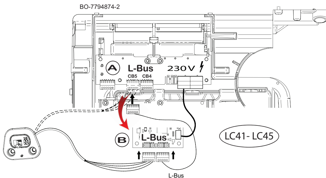
Fig.52 Collegamento scheda accessoria in caldaia
