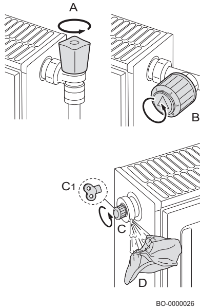
Fig.22 Deareazione impianto
