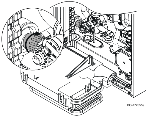
Fig.54 Scarico impianto
