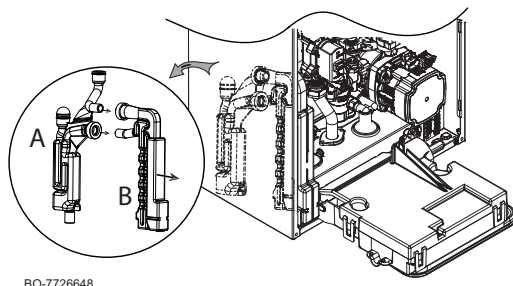
Fig.73 Smontaggio del sifone
