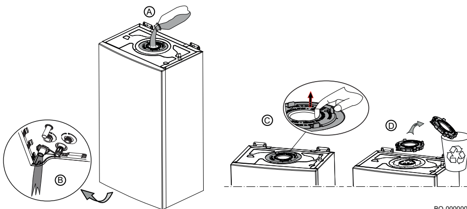
Fig.55 Modalità di riempimento del sifone prima di montare la torretta
