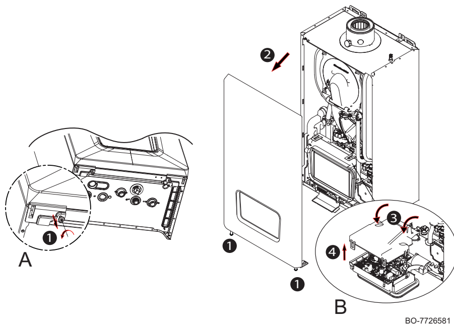
Fig.47 Accesso ai collegamenti elettrici
