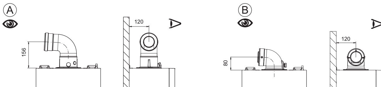
Fig.41 Tipo di scarico-aspirazione coassiale
