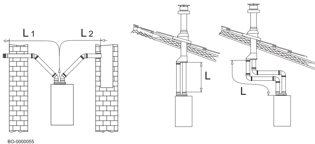
Fig.46 Esempi installazioni condotti separati
