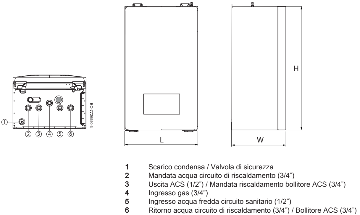
Fig.24 Dimensioni e collegamenti modello compatto
