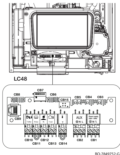
Fig.49 Collegamenti scheda di caldaia
