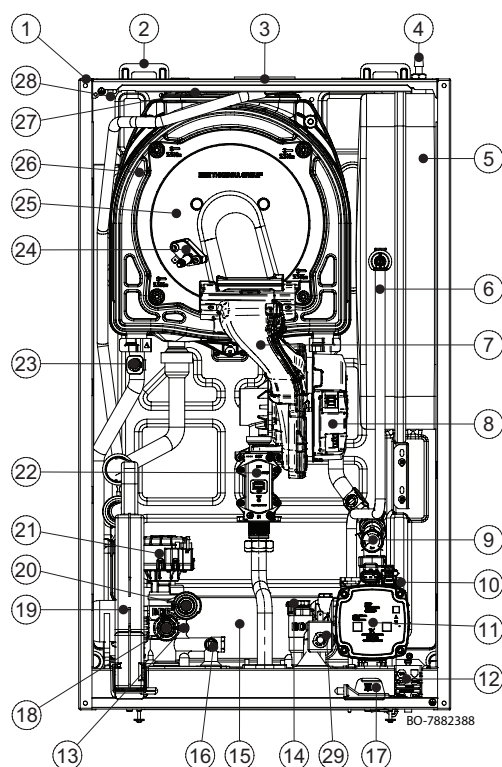
Fig.28 Descrizione componenti
