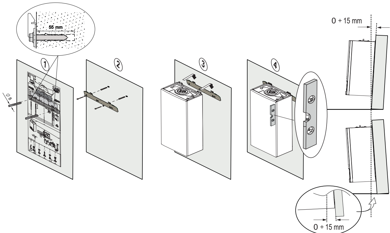
Fig.35 Installazione a parete
