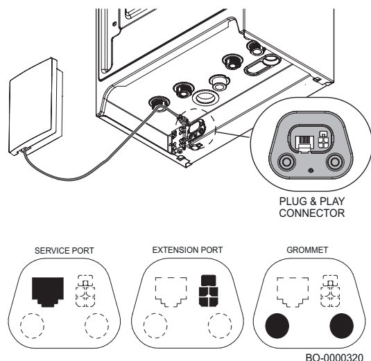
Fig.50 Posizione del connettore
