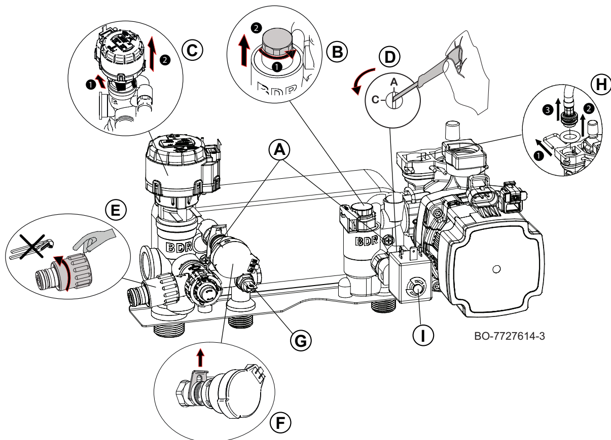
Fig.75 Particolare gruppo idraulico caldaia combinata Riscaldamento + ACS
