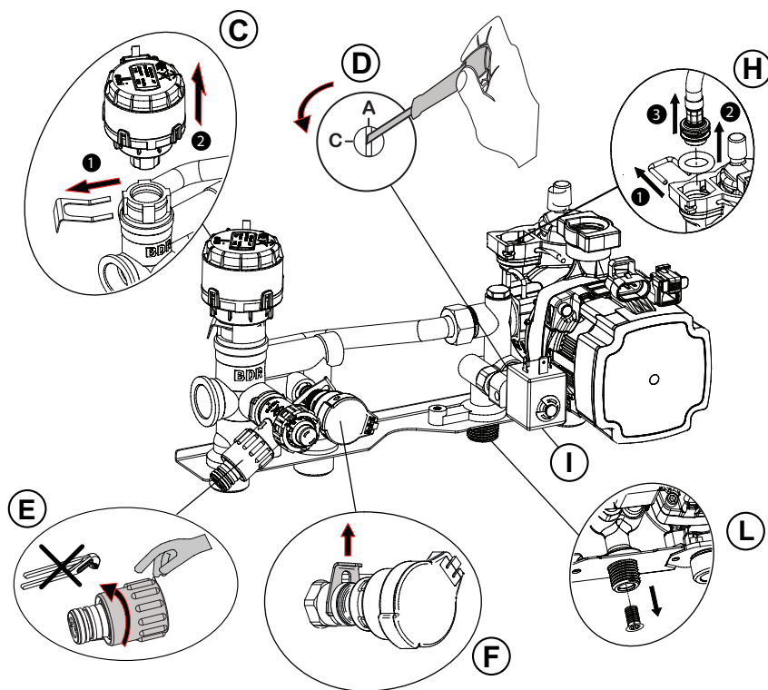
Fig.76 Particolare gruppo idraulico caldaia solo Riscaldamento con predisposizione collegamento bollitore ACS
