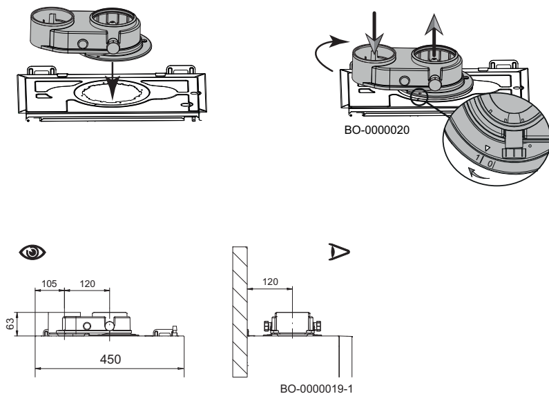
Fig.45 Installazione raccordo per condotti separati
