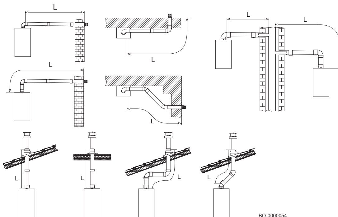
Fig.43 Esempi installazioni condotti coassiali
