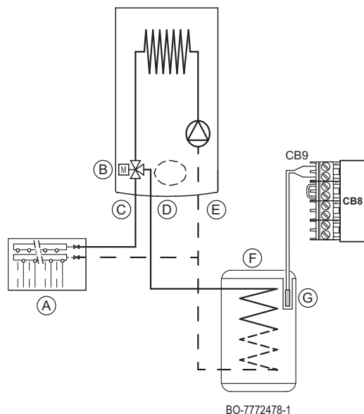
Fig.38 Connessione bollitore ACS
