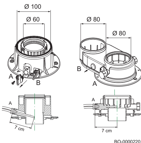
Fig.58 Tipologie di raccordi — punto di misurazione fumi
