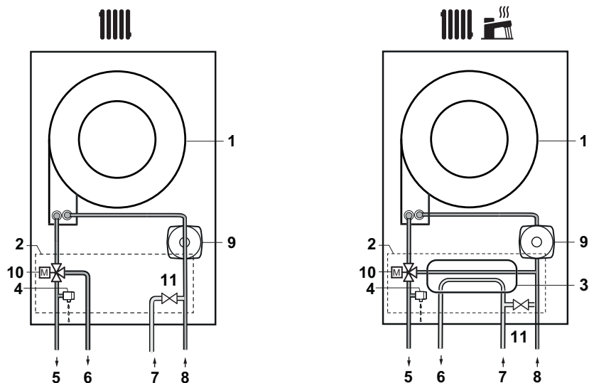
Fig.27 Schema di principio modelli solo riscaldamento e riscaldamento con Acqua Calda Sanitaria istantanea
