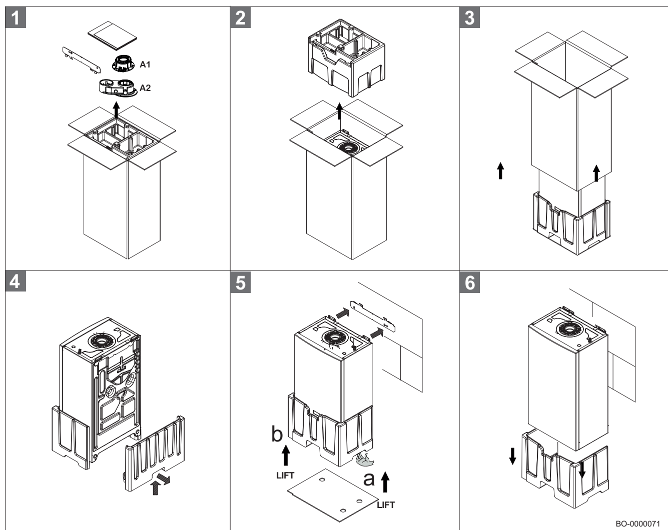
Fig.34 Procedura di disimballo
