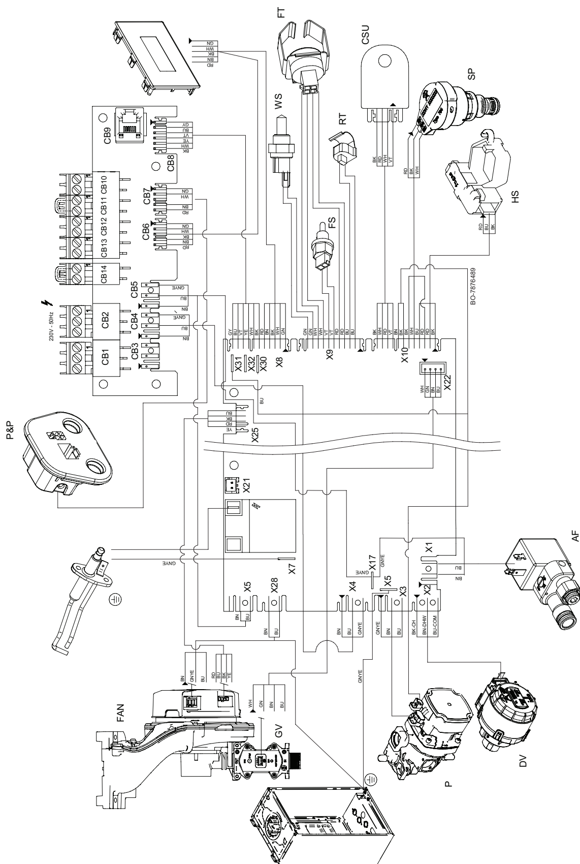
Fig.26 Schema collegamenti elettrici di caldaia
