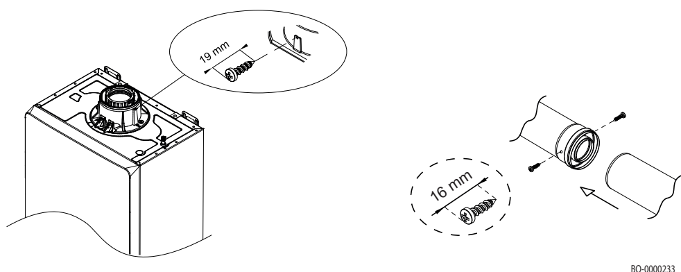
Fig.42 Fissaggio torretta fumi coassiale
