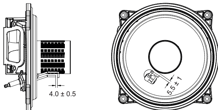
Fig.74 Distanze elettrodo
