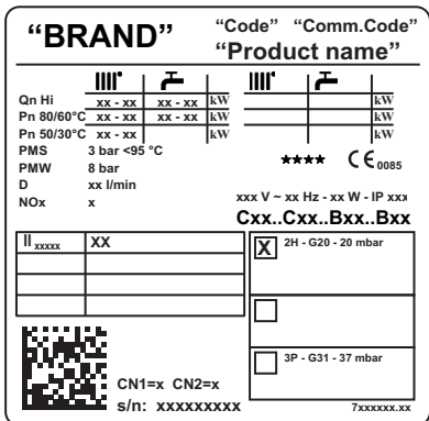
Fig.32 Targa matricola
